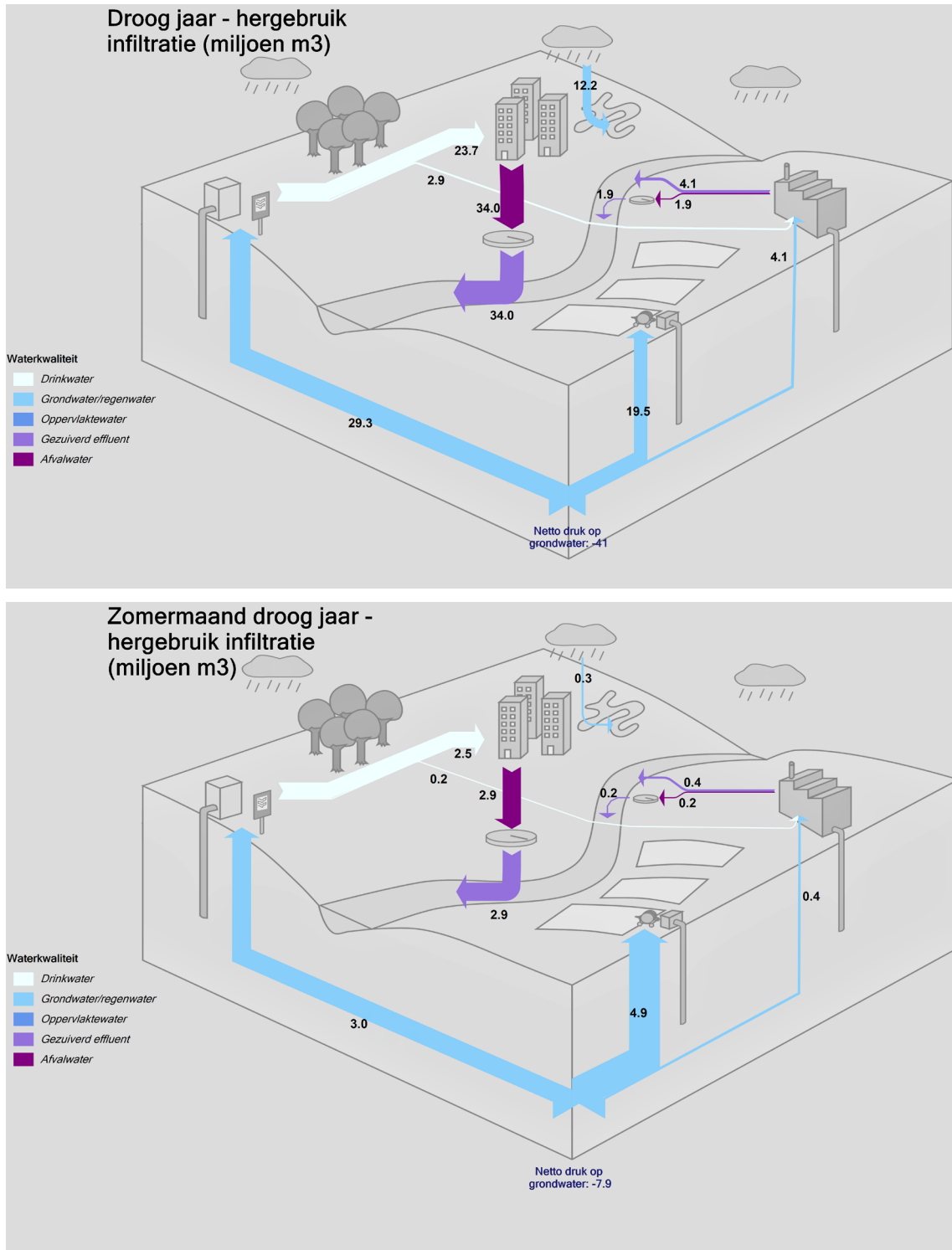
FIGUUR 3.15 SANKEY-DIAGRAMMEN VAN DE WATERSTROMEN IN EEN DROOG JAAR (BOVEN) EN DROGE ZOMERMAAND (ONDER) IN HET DERDE WATERFABRIEK-SCENARIO (RWA NAAR GRONDWATER), GEBASEERD OP HET JAAR 2019
