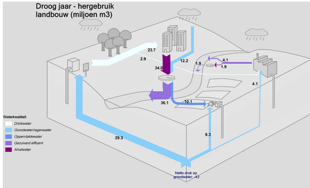
SANKEY-STROOMDIAGRAM VAN DE WATERSTROMEN IN EEN DROOG JAAR (2019), WAARBIJ EFFLUENT DEELS WORDT HERGEBRUIKT VOOR LANDBOUWDOELEINDEN
