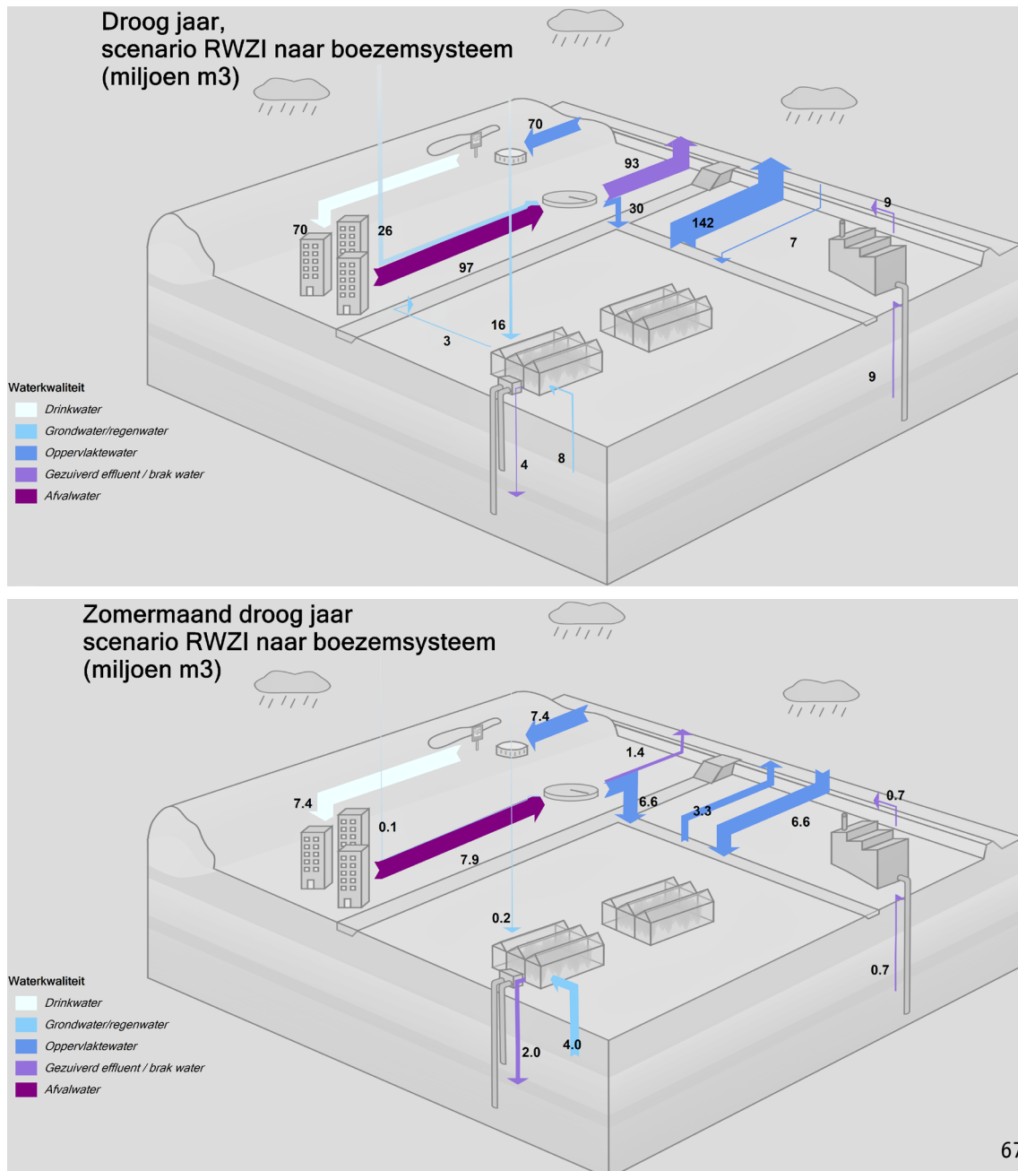
FIGUUR 4.12 SANKEY-DIAGRAMMEN VAN DE WATERSTROMEN IN EEN DROOG JAAR (2018, BOVEN) EN DROGE ZOMERMAAND IN DAT JAAR (ONDER) IN HET TWEEDE WATERFABRIEK-SCENARIO (RWZI NAAR BOEZEMSYSTEEM) IN CASUS 2
