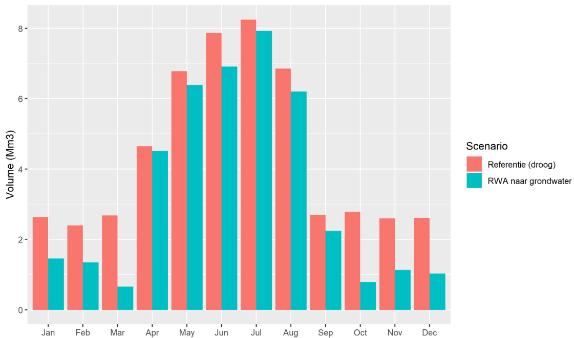
FIGUUR 3.16 TOTALE ANTROPOGENE DRUK OP HET GRONDWATER (DRINKWATER + INDUSTRIE + LANDBOUW) MINUS RWA-INFILTRATIE IN HET DERDE WATERFABRIEK- SCENARIO (RWA NAAR GRONDWATER), VERGELEKEN MET DE DROGE REFERENTIESITUATIE
