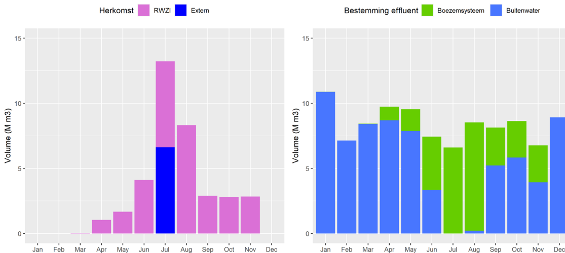
FIGUUR 4.14 LINKS: HERKOMST VAN HET AANGEVOERDE OPPERVLAKTEWATER IN HET TWEDE WATERFABRIEK-SCENARIO (RWZI NAAR BOEZEMSYSTEEM) IN CASUS 2. RECHTS: BESTEMMING VAN HET EFFLUENT VAN RWZI'S GROOTE LUCHT, NIEUWE WATERWEG EN HARNASCHPOLDER
