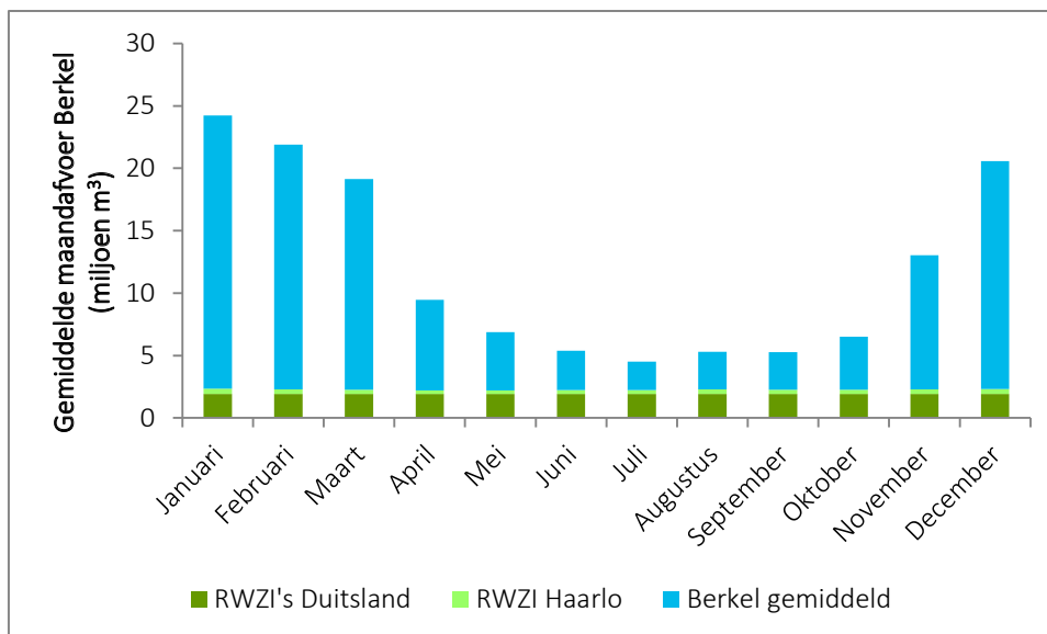
Figuur 13, Gemiddelde maandaafvoer van de rivier de Berkel. De Berkel is de belangrijkste rivier in het casusgebied en speelt een belangrijke rol in de lokale drinkwatervoorziening. Een deel van het Berkel water wordt opgemaakt door Duits RWZI water. Daarnaast loost ook RWZI Haarlo effluent op de Berkel. Op maandbasis vormt het aandeel effluent al bijna de helft van de totale afvoer in de zomer. Voor inzicht in de dagafvoer en basisafvoer, zie figuur 12.
