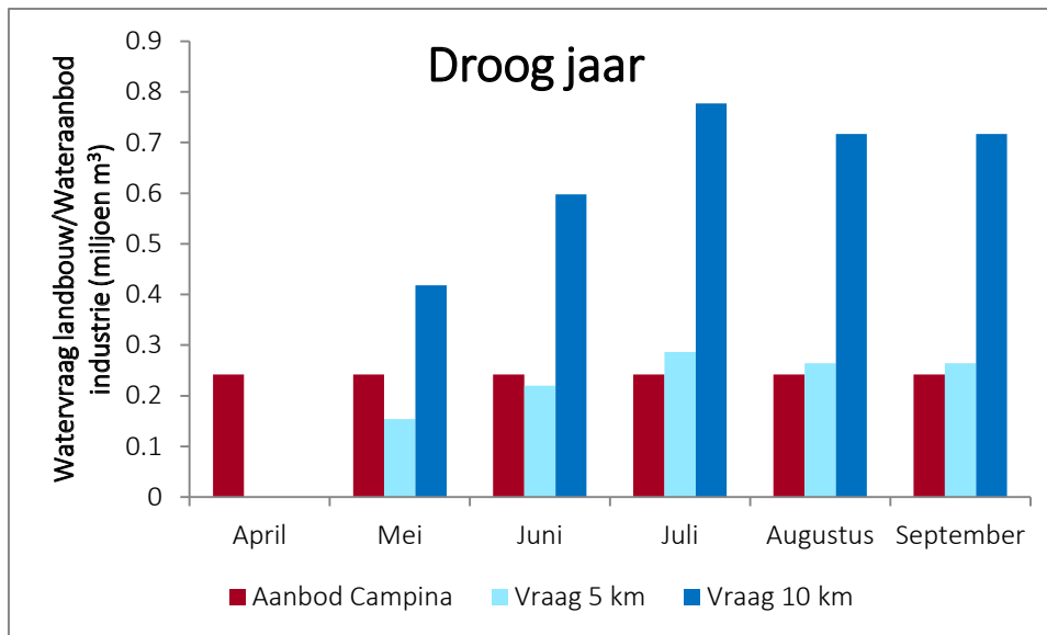
Figuur 19, Watervraag van landbouw en wateraanbod van Campina in scenario 2. In dit scenario is gebruik gemaakt van 2 zones rondom de Campina locatie. Een tot 5 km vanaf de vestiging van Friesland Campina Domo in Borculo en eentje tot 10 km vanaf de vestiging (figuur 20). In dit scenario is aangenomen dat de vraag evenwijdig verdeeld is over het casusgebied omdat niet alle gegevens van grondwater onttrekkers uit het LGR compleet bleken.
