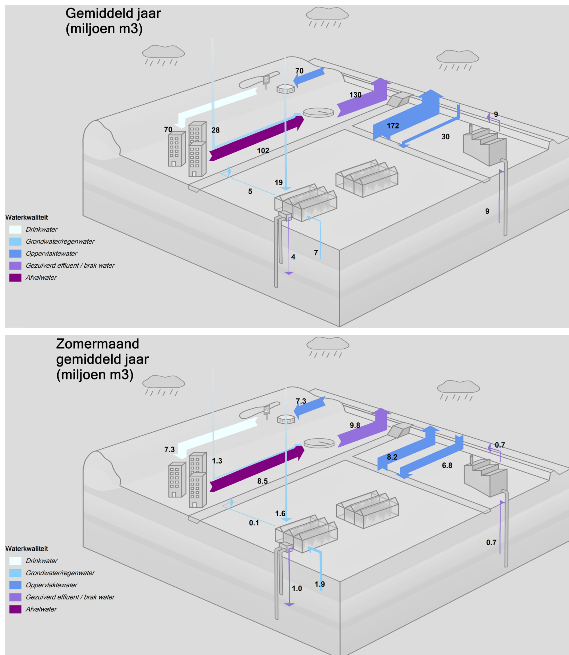
FIGUUR 4.2 SANKEY-DIAGRAMMEN VAN DE WATERSTROMEN VAN HET ANTHROPOGENE WATERSYSTEEM IN EEN GEMIDDELD JAAR (BOVEN) EN GEMIDDELD ZOMERMAAND (ONDER) IN CASUS 2, GEBASEERD OP DE PERIODE 2015-2019
