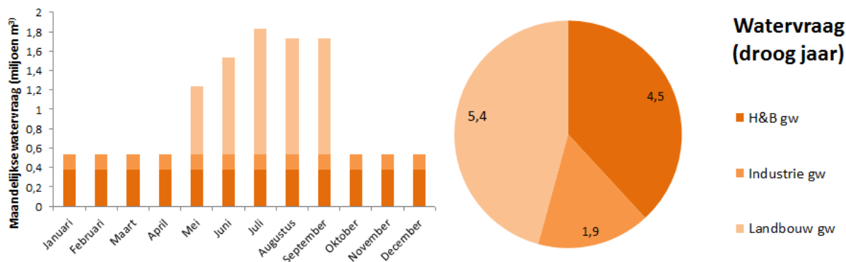
Figuur 15, Watervraag van huishoudens en bedrijven (H&B), landbouw en industrie gedurende een droog jaar op basis van de verschillende beschikbare waterbronnen. Ongeveer al het gebruikte water in het casusgebied wordt gewonnen uit grondwater (oranje). Jaartotaal van de vraag in het casusgebied in een droog jaar is 11,8 miljoen m 3 , oftewel 34 mm.
